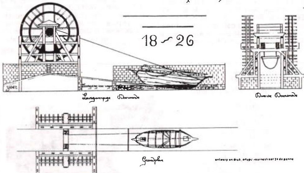
Technisch detail van de in 1826 afgebroken windas of „winde” op de samenvloeiing van de IJzer en de Lovaart, ter hoogte van het gehucht Fintele („windeele”).
